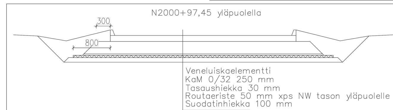
Veneluiskan periaatempoikkileikkaukset 1:50
