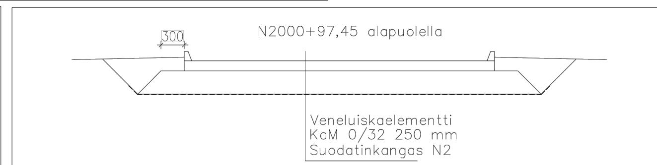
Veneluiskan periaatempoikkileikkaukset 1:50
